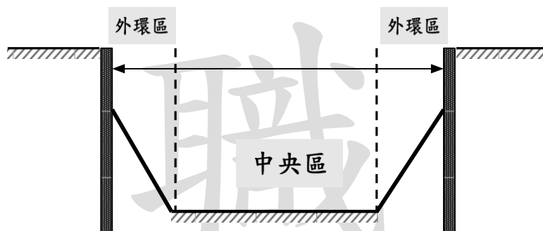
圖 2 基地中央區土方開挖
