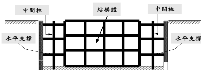
圖 3 施築中央區結構體
