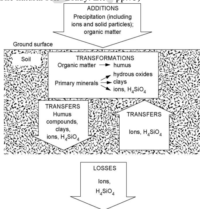
圖 4-4 土壤形成的過程
