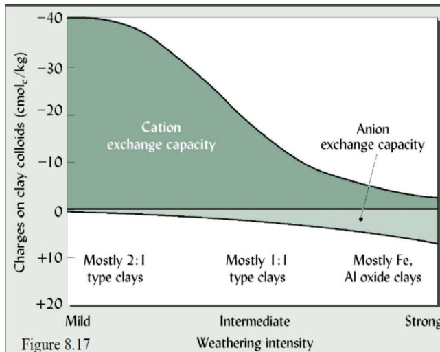
圖 1 土黏土風化對土壤 CEC 的關係
