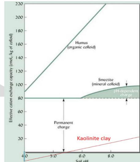
圖 2 pH 值對 CEC 的影響圖
