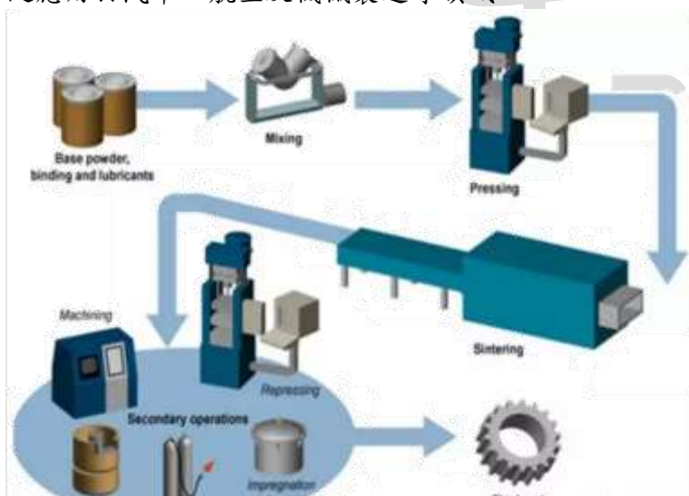
粉末冶金製程的步驟示意圖
