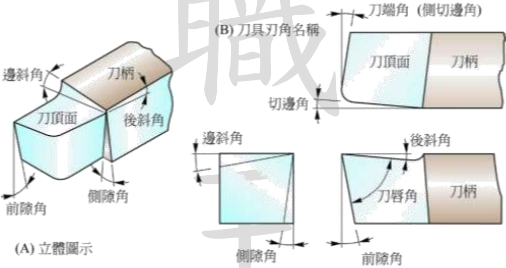
圖 高速鋼車刀刀角
